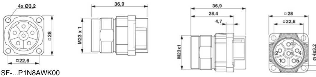
Installation dimensions SF-...P1N8AWK00
